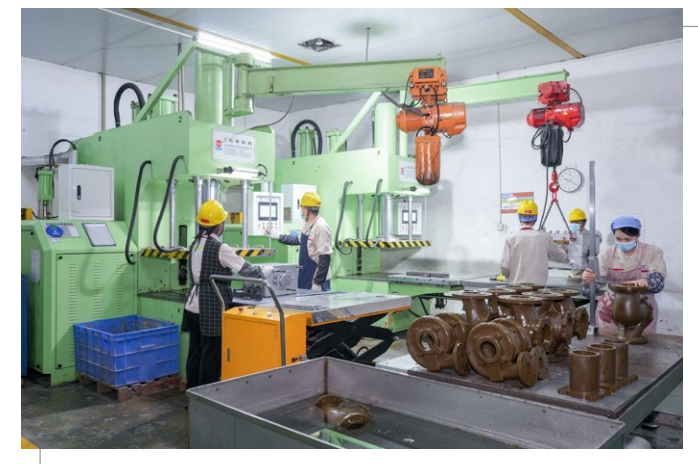
蜡模制作 Wax pattern production
